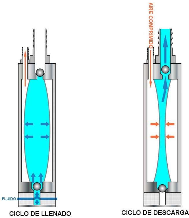
Figura 1 – Funcionamiento de la Bomba de Vejiga
