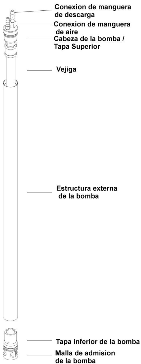
Figura 2 – Montaje Básico* de Bomba de Vejiga Portátil
