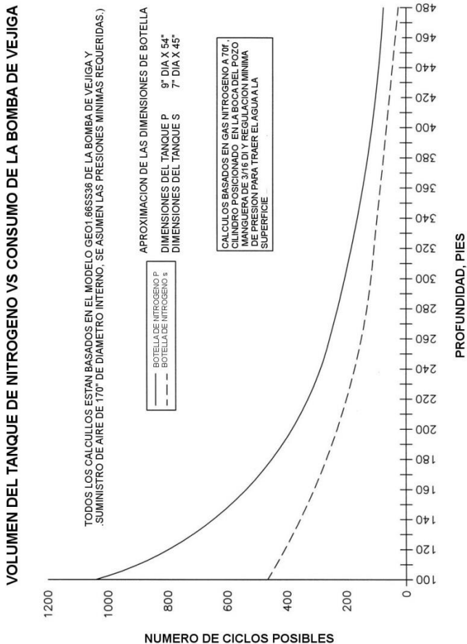
Figura 5 – Volumen del Tanque vs. Consumo de la Bomba
