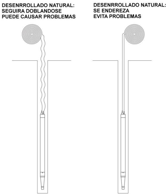
Figura 3 – Método de enrollado inverso
