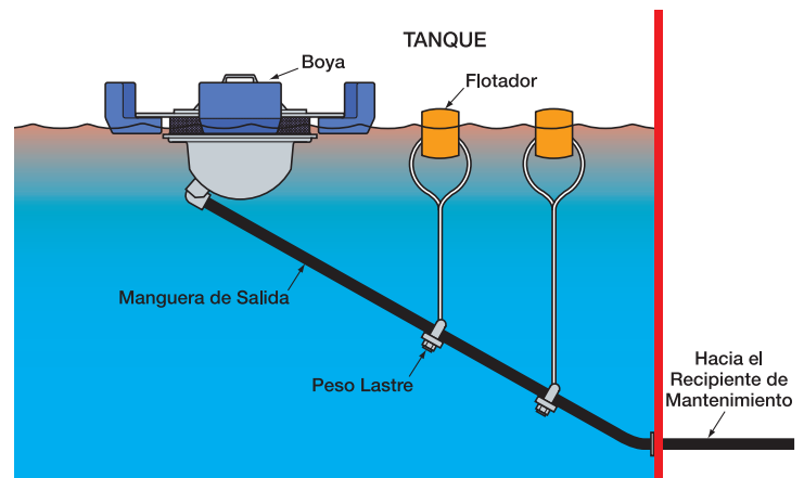
Diagrama de Operación de la Geotech Gravity Feed Filter Scavenger
